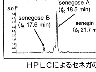
HPLCによるセネガの成分比較
